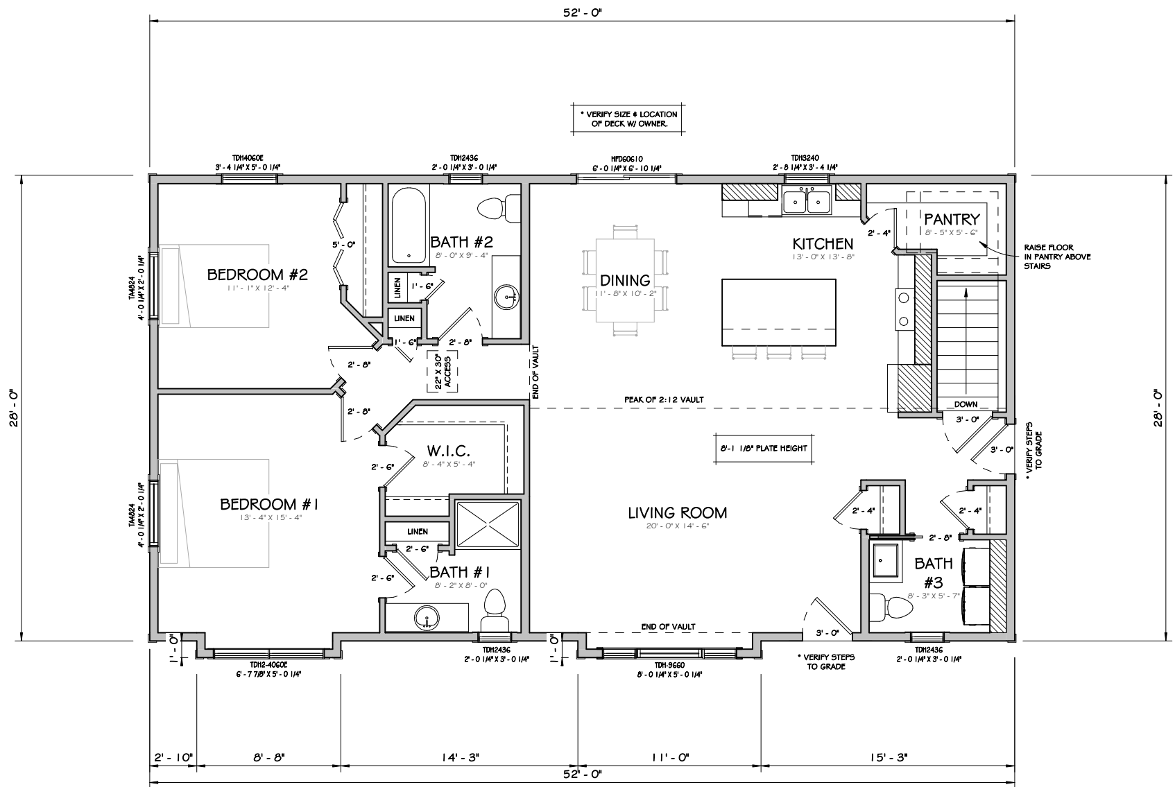
1 MAIN LEVEL A3 1/8" = 1'-0"
