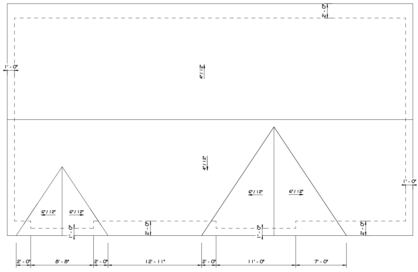
2 ROOF PLAN A5 1/8" = 1'-0"
