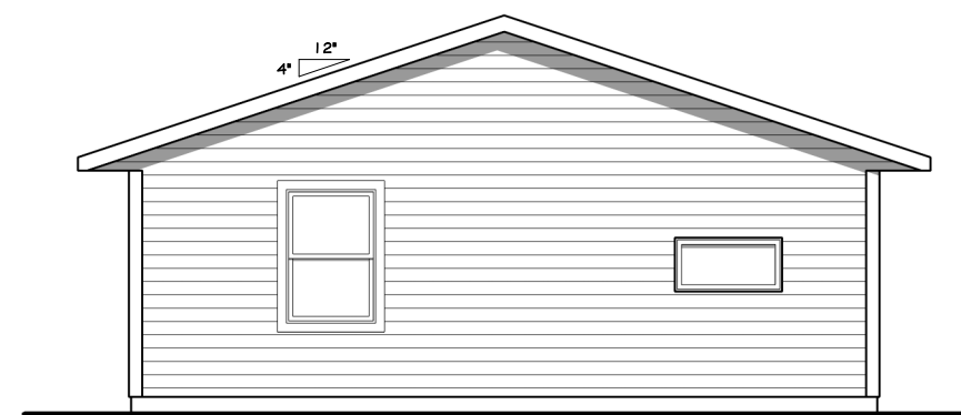
4 LEFT ELEVATION AI 1/8" = 1'-0"
